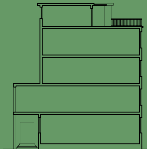
SEZIONE A-A'
